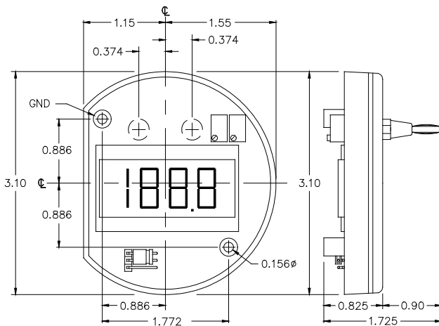
MODULE DIMENSIONS
